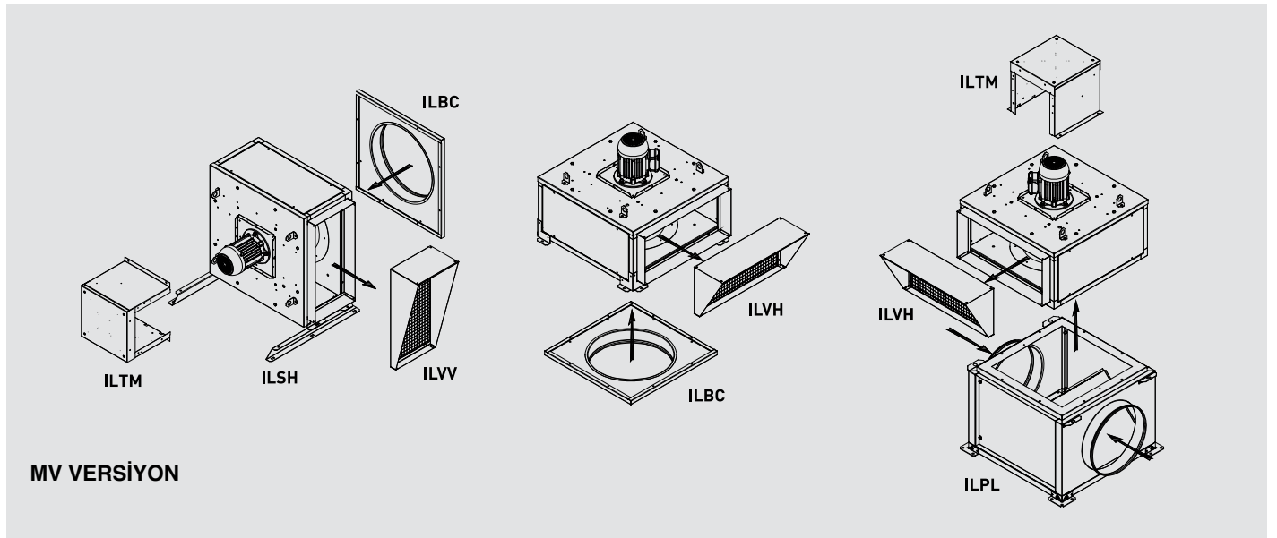
ILSH Motorun yatay konumda olduğunda montaj desteği
