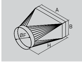
ILRC Çıkış dairesel kanal bağlantı flanşı
